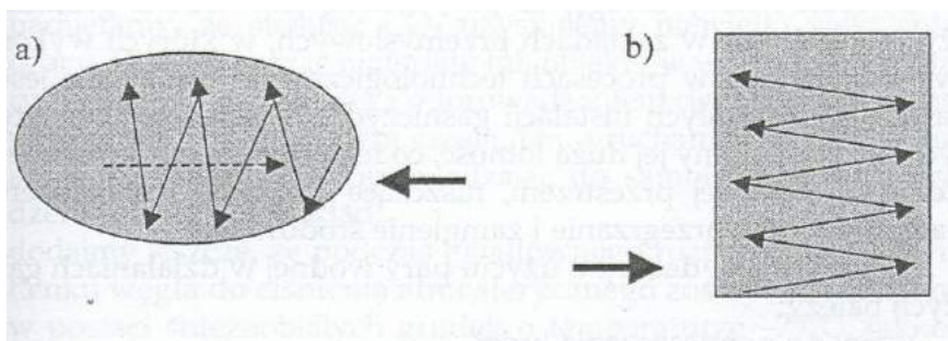
Rysunek nr 10.9. Gaszenie pianą: a) cieczy rozlewającej się, b) konstrukcji pionowych 156
