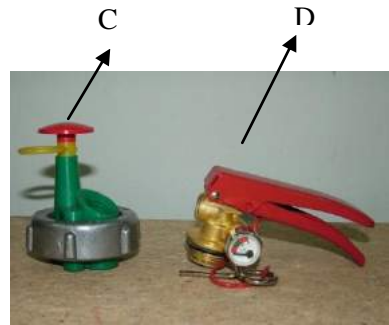
Fotografia nr 3.25 C. Głowica gaśnicy z ładunkiem CO 2 D. Zawór gaśnicy pod stałym ciśnieniem
