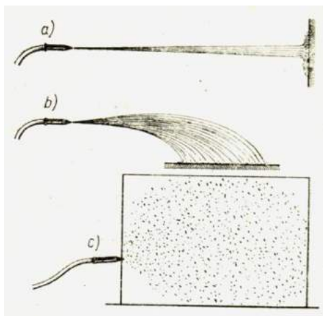
Rysunek nr 10.4. Działanie prądów wody: a – zwartego (punktowe), b – kroplistego (powierzchniowe), c – mgłowego (przeźrzennego) 139
