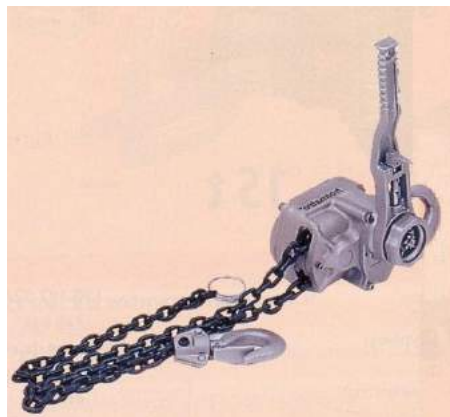
Fotografia nr 3.22. Wyciągarka łańcuchowa 51
